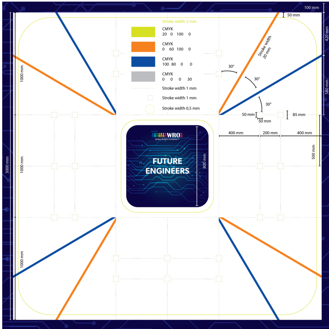
Ábra: A versenypálya pontos méretei
