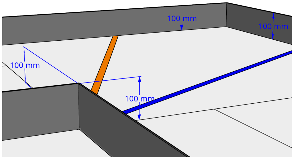
Ábra: A külső és belső falak magassága
